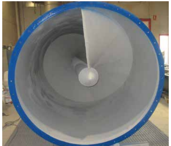
Espiras reforzadas y atornilladas en acero antidesgaste de fácil recambio.
